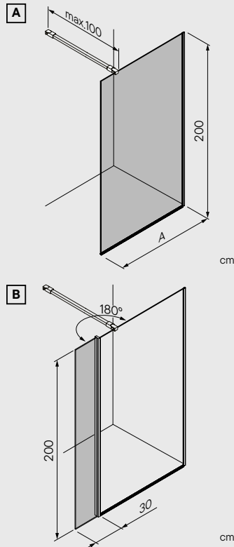
Cristal fijo Fixed panel Verre fixe
