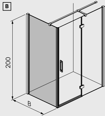
Fijo lateral Fixed side panel Fixe latéral
