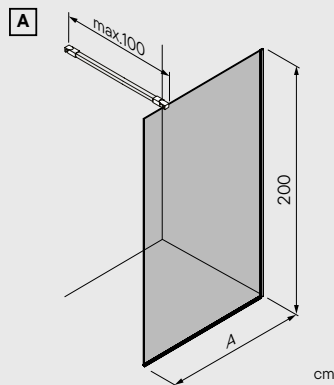
Cristal fijo Fixed panel Verre fixe
