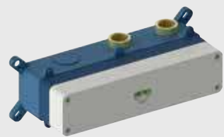
sanybox para monomando horizontal 2 vías mural Horizontal wall-mounted mixer 2 ways sanybox sanybox pour mitigeur mecanique horizontal 2 voies mural p. 65
