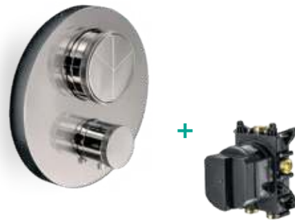
E176633-110 εξωτερικό τμήμα Inox Finish E134001 κιτ εντοιχισμού Θερμοστατικός μίκτης εντοιχισμού 3 εξόδων και κιτ εντοιχισμού
